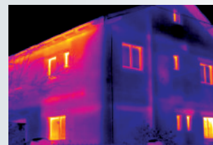
Scoprire le perdite di energia negli edifici: individuare e rappresentare immediatamente i ponti termici in una facciata o in un edificio.
